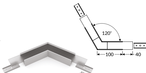
Connecteur d'angle 120°
