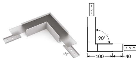
Connecteur d'angle 90°
