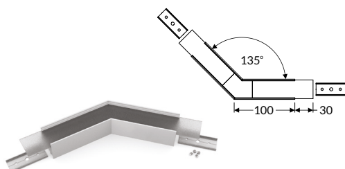
Connecteur d'angle 135°
